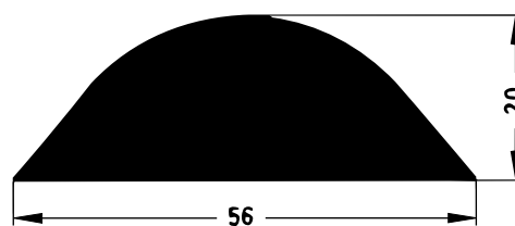
Art. 832840 RAU-SIK 8726 50±5° Shore A
