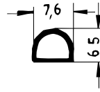
Art. 832531 RAU-SIK 8963 50±5° Shore A
