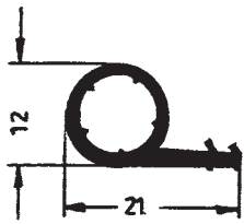
Art. 832981 RAU-SIK 8360 60±5° Shore A
