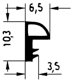
Art. 832161 RAU-SIK 8110 40±5° Shore A
