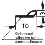
Art. 851610 RAU-SIK 8150 60±5° Shore A
