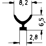
Art. 835360 RAU-SIK 8360 60±5° Shore A
