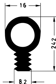
Art. 833361 RAU-SIK 8190 50±5° Shore A
