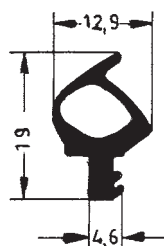
Art. 834123 RAU-SIK 8153 60±5° Shore A
