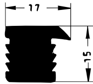
Art. 834891 RAU-SIK 8277 60±5° Shore A
