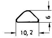
Art. 836340 RAU-SIK 8318 60±5° Shore A
