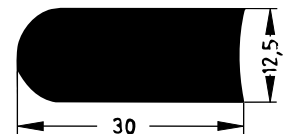
Art. 832410 RAU-SIK 8128 55±5° Shore A
