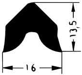
Art. 833111 RAU-SIK 8361 60±5° Shore A
