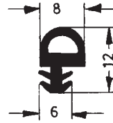
Art. 834143 RAU-SIK 8220 55±5° Shore A
