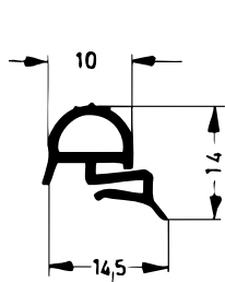
Art. 833181 RAU-SIK 8318 60±5° Shore A
