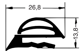
Art. 834351 RAU-SIK 8134 60±5° Shore A
