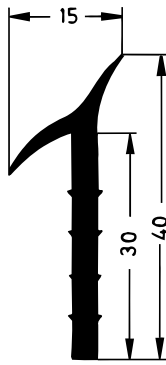
Art. 834760 RAU-SIK 8760 70±5° Shore A
