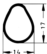
Art. 833921 RAU-SIK 8367 60±5° Shore A
