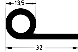
Art. 834130 RAU-SIK 8190 50±5° Shore A
