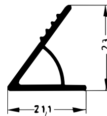
Art. 834352 RAU-SIK 8360 60±5° Shore A
