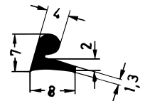
Art. 832330 RAU-SIK 8128 55±5° Shore A
