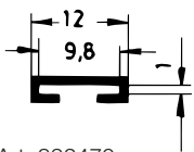
Art. 832470 RAU-SIK 8128 55±5° Shore A
