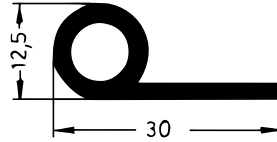
Art. 832181 RAU-SIK 8220 55±5° Shore A
