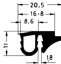
Art. 836020 RAU-SIK 8360 60±5° Shore A
