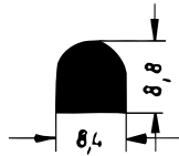
Art. 834341 RAU-SIK 8360 60±5° Shore A
