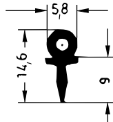
Art. 832041 RAU-SIK 8318 60±5° Shore A
