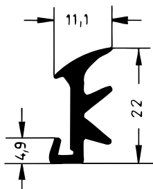
Art. 832231 RAU-SIK 8725 50±5° Shore A
