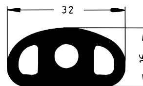
Art. 832031 RAU-SIK 8367 60±5° Shore A
