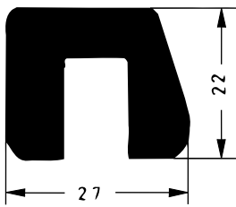
Art. 832441 RAU-SIK 8280 33±5° Shore A
