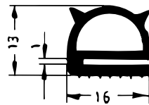
Art. 832791 RAU-SIK 8963 65±5° Shore A
