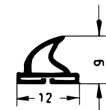
Art. 833391 RAU-SIK 8318 60±5° Shore A
