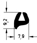
Art. 832071 RAU-SIK 8318 60±5° Shore A
