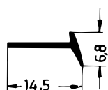
Art. 834980 RAU-SIK 8360 60±5° Shore A
