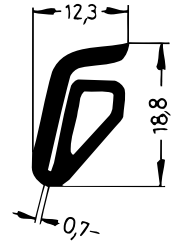
Art. 832091 RAU-SIK 8238 50±5° Shore A
