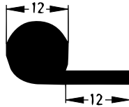
Art. 832040 RAU-SIK 8280 33±5° Shore A
