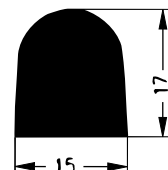
Art. 832460 RAU-SIK 8280 33±5° Shore A
