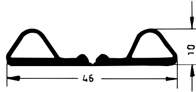
Art. 833911 RAU-SIK 8367 60±5° Shore A
