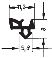
Art. 834063 RAU-SIK 8318 60±5° Shore A
