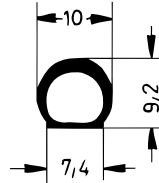
Art. 832291 RAU-SIK 8855 70±5° Shore A
