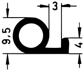
Art. 833300 RAU-SIK 8128 55±5° Shore A
