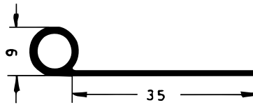
Art. 832420 RAU-SIK 8360 60±5° Shore A
